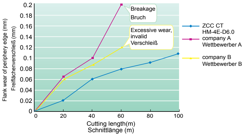
Cycloid machining of end mill Zyklische Bearbeitung
